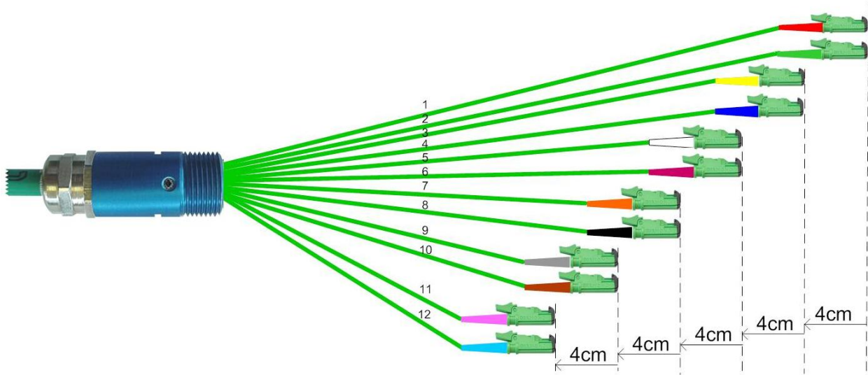
Aufteiler 12-fasrig doppelt gestuft/ Forcation 12 Fibres / Eclateur 12 Fibres
