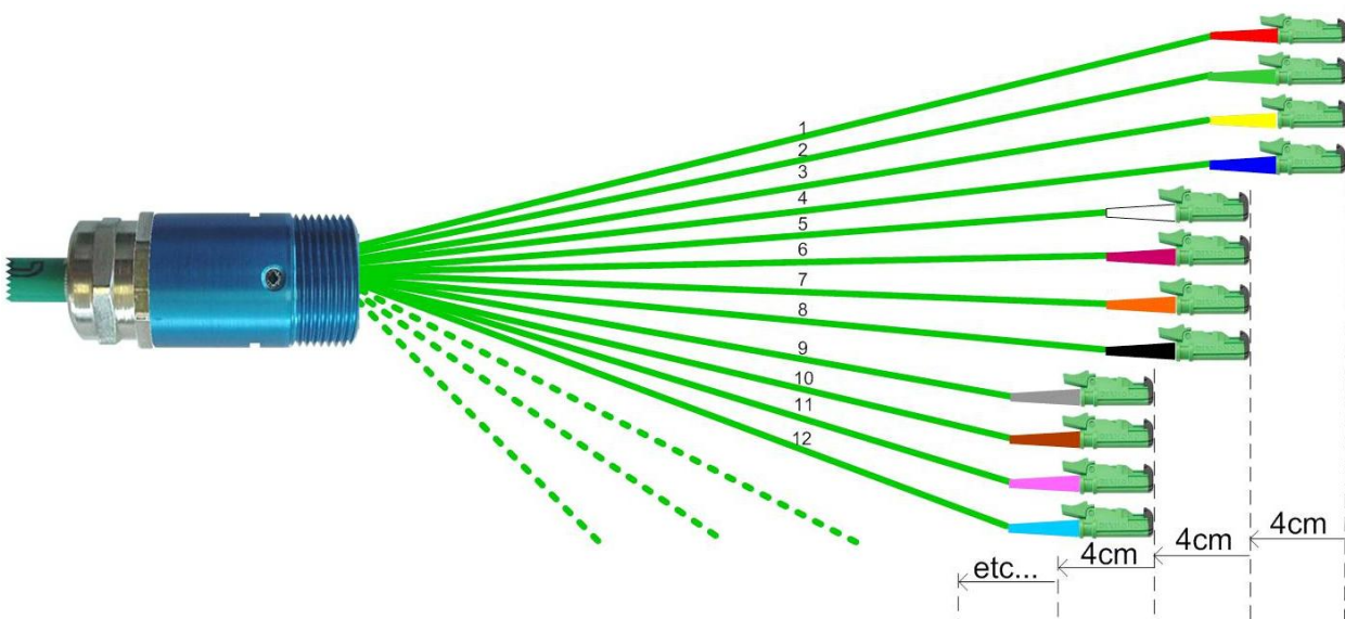
Aufteiler 24-fasrig vierfach gestuft/ Forcation 24 Fibres / Eclateur 24 Fibres
